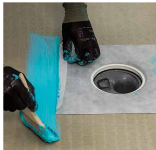
6. Sivele laipan reuna-alueen vahvikangas Kiilto Kerafiberillä.
