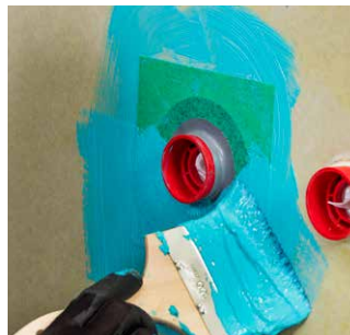
10. Hierrä Kiilto Läpivientvahvike märkään Kiilto Kerafiberiin ja sivele yli.
